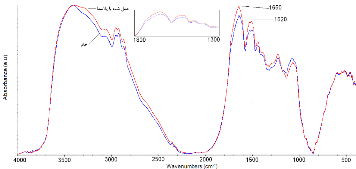
شکل ۷: طیف FTIR نمونه‌های پشم خام و عمل شده با پلازما (۵۰ وات، ۳۰۰ ثانیه).
