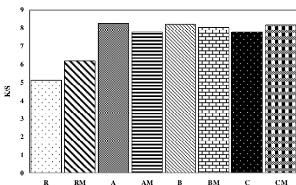
شکل ۵: تاثیر دندانده بر قدرت رنگی نمونه‌های خام (R) و پلازما شده (A,B,C) در pH=۵، دمای ۸۰ °C و زمان ۶۰ دقیقه، (نمونه دندانده شده با (M) مشخص شده‌اند).
