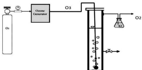
شکل ۱: شمایی راکتور و تجهیزات مورد نیاز.
