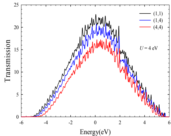
شکل ۲. (رنگی در نسخه الکترونیکی) نمودار ضریب عبور الکترونی برحسب انرژی برای یک نانو بلور با سطح مقطع 7 \times 7 شامل یک بار مثبت الکتریکی در سه جایگاه متفاوت در سطح مقطع. نانو بلور در راستای طول نامتناهی فرض شده است.
