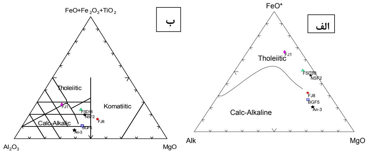
شکل ۱۰ الف - نمودار AFM جهت تعیین سری ماگمایی سنگ‌های آذرین مافیک مجموعه‌ی افیولیتی. جهت تعیین سری ماگمایی این سنگ‌ها در میدان بازالت‌های پشته‌های میان اقیانوسی تصویر شده است. ترکیب شیمیایی سنگ‌های آذرین مافیک در
