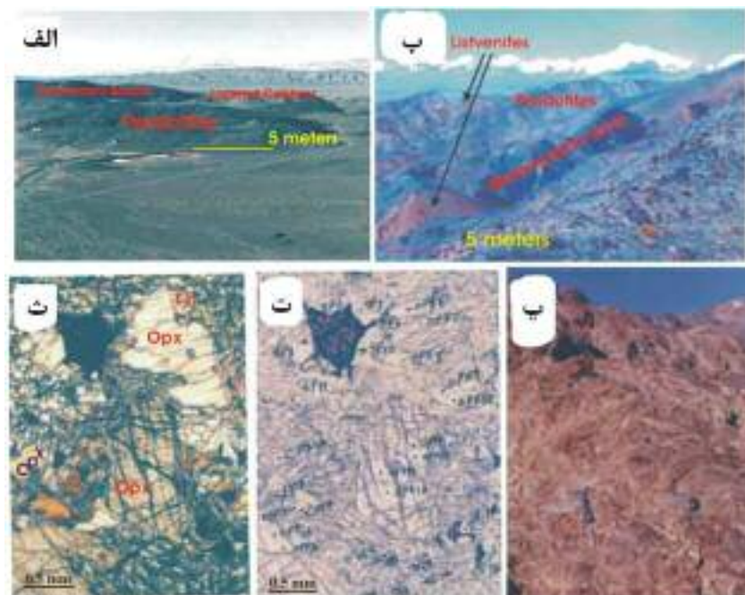
شکل ۴ الف- دنباله‌ی پریدوتیت و گابرو لایه‌ای در حدود ۲ کیلومتری جنوب غرب سولابست (دید به سمت جنوب غربی). ب- لیستونیتی شدن پریدوتیت‌ها در حدود ۱۰ کیلومتری شمال تا شمال غربی گزیک (دید به سمت غرب). پ - بقایای بیضوی شکل پریدوتیت در زمینه‌ی لیستونیت در ۲ کیلومتری شمال شرقی گزیک (دید به سمت جنوب غرب). ت - تصویر میکروسکوپی اسپینل هارزبورژیت (TDF4) و نقاط آنالیز شده‌ی کانی‌های آن (NPL). ث- الیوین، اورتوپيروكسن و دیوپسید در همان نمونه با یک بافت پورفیروکلاستیکی (XPL). Ol = Olivine, Opx = Orthopyroxene, Cpx = Clinopyroxene, Sp = Spinel
