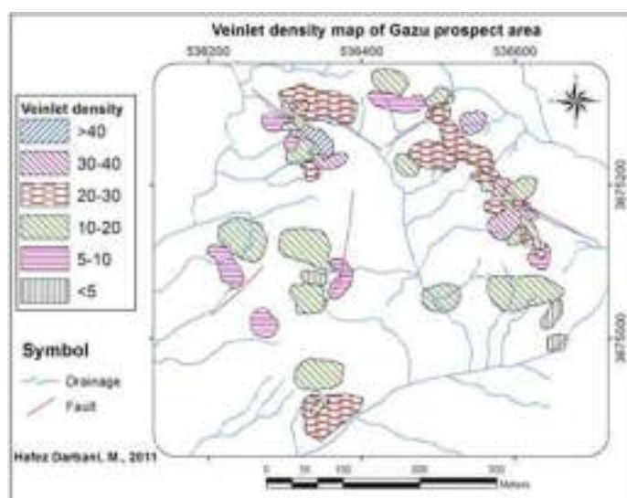
شکل ۷ نقشه تراکم رگچه‌ی گستره‌ی پی‌جویی گزو.
