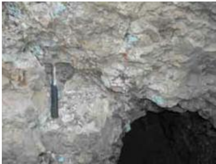
شکل ۲ حضور مالاکیت وسیع در سطح تونل‌های قدیمی.
