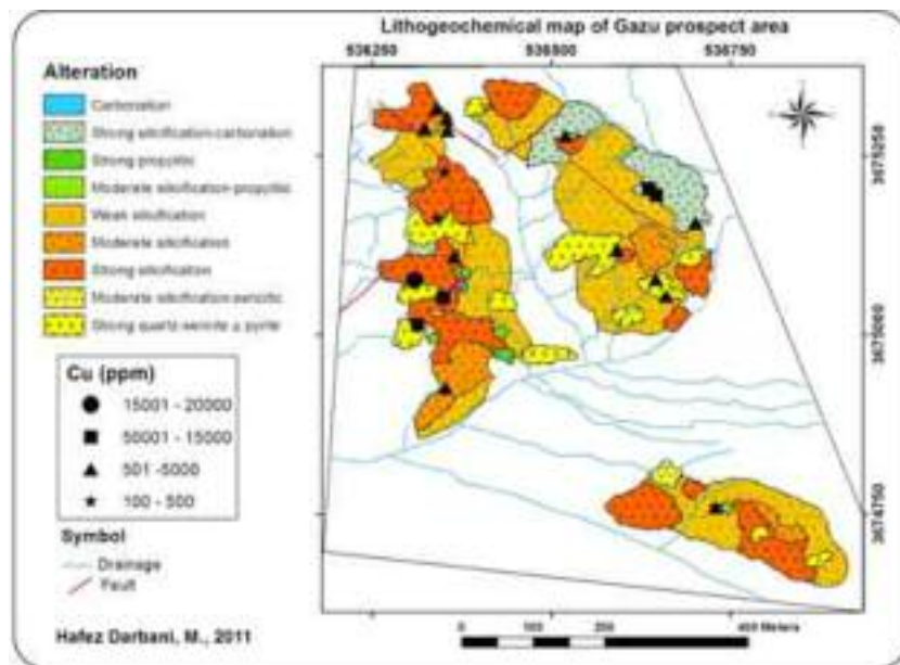
شکل ۱۴ الف- نقشه‌ی ژئوشیمی خردسنگی عنصر مس، گستره‌ی پی جویی گزو.
