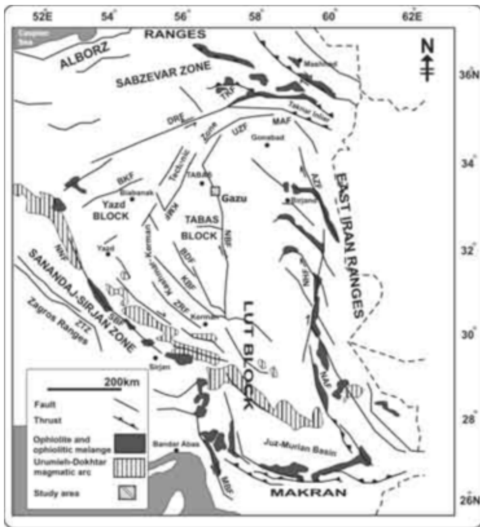
شکل ۱ نقشه‌ی تقسیمات ساختاری مرکز و شرق ایران و موقعیت منطقه‌ی مورد بررسی بر روی آن (برگرفته از [۵،۱] با تغییرات پس از [۶]). = MAF = گسل میناب، = NAF = گسل نصرت آباد، = NBF = گسل نایبند، = NHF = گسل نهبندان، = NNF = گسل ناین، = SBF = گسل شهربابک، = TKF = گسل تکنار، = UZF = گسل ازبک کوه، = ZRF = گسل زرنند، = ZTZ = زون تراستی زاگرس.
