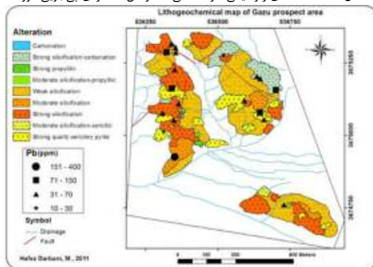
شکل ۱۴ ب- نقشه‌ی ژئوشیمی خردسنگی عنصر سرب، گستره‌ی پی جویی گزو.
