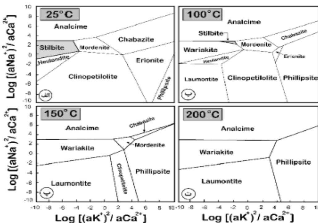
شکل ۱۱ نمودار تغییرات محدوده پایداری زئولیت‌ها با افزایش دما (الف تا ت) [۱۹].
