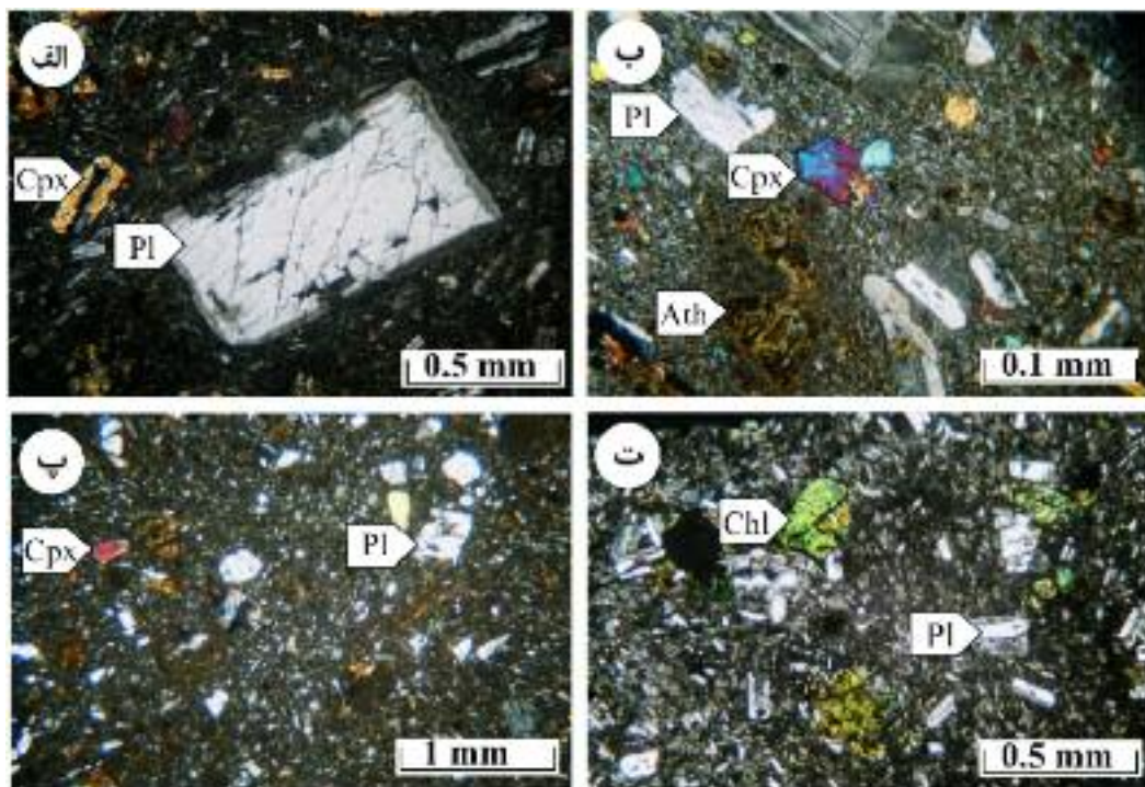
شکل ۳ تصاویر میکروسکوپی از واحدهای سنگی مورد بررسی. الف- فنوکریست پلاژیوکلاز به همراه اوژیت در زمینه‌ی ریز بلوری تراکی‌اندزیت (XPL)، بافت ریز بلوری پورفیری در تراکی‌اندزیت با حضور پلاژیوکلاز و اوژیت و دگرسانی اولیوین به آنتوفیلیت (XPL)، پ - پلاژیوکلاز و کلینوپيروكسن در زمینه‌ی ریزدانه واحد توفی (XPL)، تبدیل‌شدگی فرومنیزین‌ها به کلریت در واحد توفی با بافت ریز بلوری (XPL).
