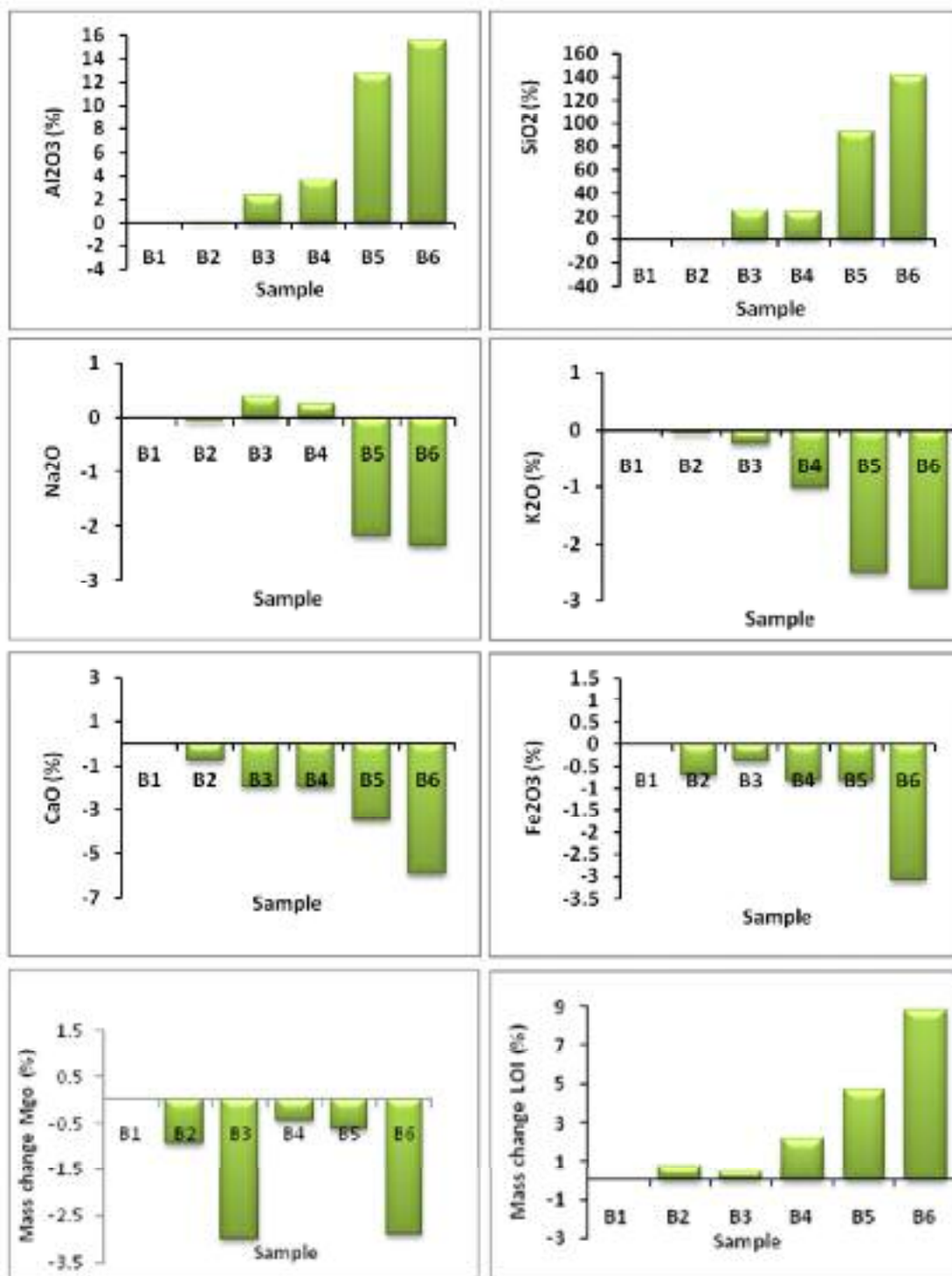
شکل ۶ نمودار تغییرات جرم اکسیدهای اصلی در طی نیم‌برداری (B1-B6).
