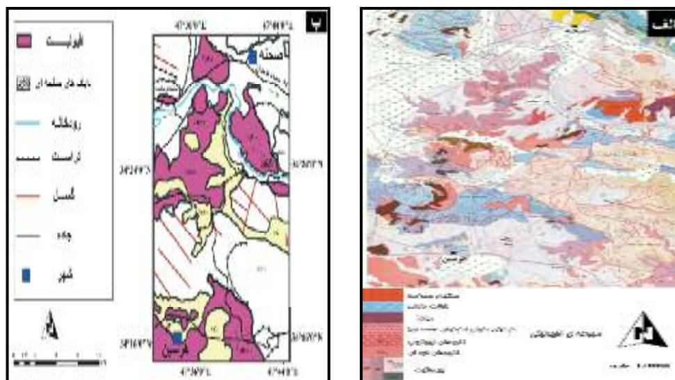
شکل ۲ الف) نقشه‌ی زمین‌شناسی منطقه‌ی مورد بررسی که در آن محل پراکندگی دایک‌ها مشخص شده است. (ب) تغییراتی اقتباس از [۱۹].
