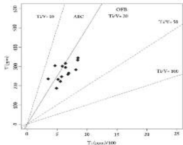
شکل ۱۱ نمودار تعیین محیط زمین‌ساختی [۳۱].
