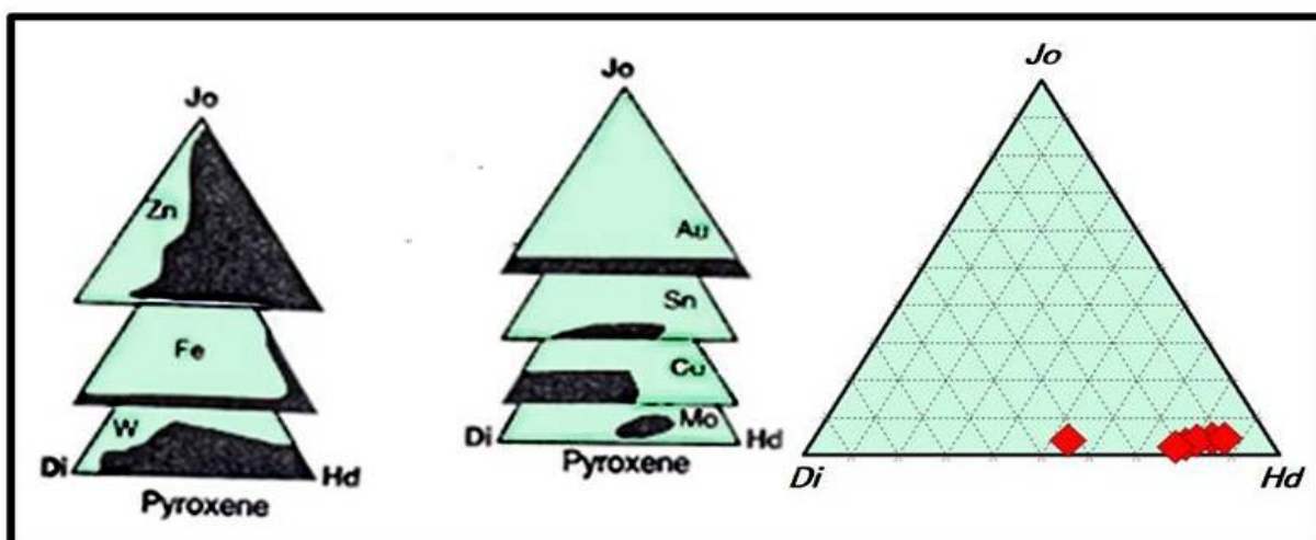
شکل ۶ نمودار توزیع ترکیب تجزیه‌های نقطه‌ای کمی کلینوپیروکسن‌ها و مقایسه آن با اسکارن‌های جهان [۴] (Di: diopside; Hd: johannsenite:hedenbergite).
