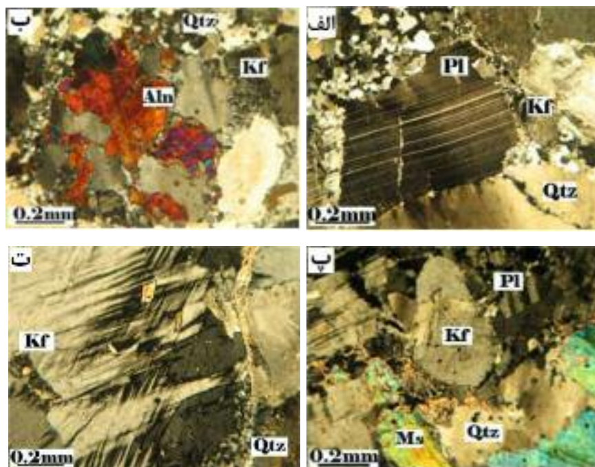
شکل ۳ تصاویر میکروسکوپی نمونه‌های پگماتیتهای منطقه در نور XPL. الف) گرانودیوریت پگماتیتهای با کوارتزهای ساب‌گرن شده و پلاژیوکلاز با ماکل‌های خمیده. ب) حضور آلانیت در پگماتیت‌های منطقه. پ) مونزودیوریت پگماتیتهای منطقه. ت) ارتوکلاز دگرشکل شده حاوی ماکل تارتن (میکروکلین) در برخی قسمت‌های بلوره‌های آن. Pl: پلاژیوکلاز، Kf: فلدسپار پتاسیم، Qtz: کوارتز، Ms: موسکوویت، Aln: آلانیت.
