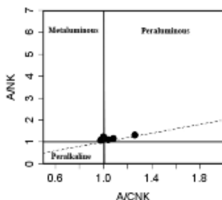
شکل ۵ نمودار تغییرات A/CNK نسبت به [A]_{NK}/20 که نشان دهنده‌ی طبیعت مت‌آلومین تا پرآلومین نمونه‌های مورد مطالعه است.
