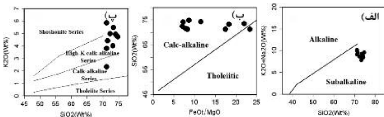
شکل ۶ تعیین سری ماگمایی: الف) موقعیت نمونه‌های مورد بررسی در نمودار مجموع اکسیدهای قلیایی نسبت به SiO_2 [۲۱] نمونه‌ها در سری نیمه قلیایی قرار می‌گیرند. ب) موقعیت نمونه‌های مورد بررسی در نمودار FeO_t/MgO نسبت به SiO_2 [۲۲] نمونه‌ها در سری آهکی-قلیایی قرار می‌گیرند. پ) موقعیت نمونه‌های مورد بررسی در نمودار SiO_2 نسبت به K_2O [۲۳]، اکثر نمونه‌ها در گستره‌ی آهکی-قلیایی پتاسیم متوسط تا بالا قرار می‌گیرند.
