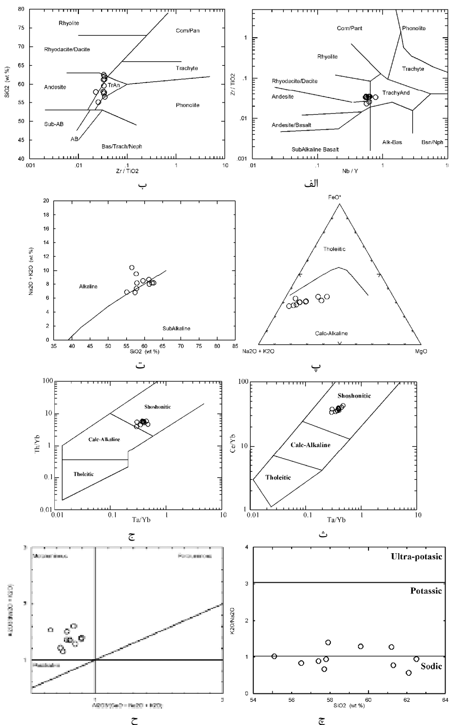
شکل ۴ نمودارهای الف و ب تعیین کننده نام سنگ [۱۶]، پ، ت، ث و ج تعیین کننده سری ماگمایی [۱۷-۱۹، ۲۱]، چ میزان پتاسیم [۲۲]، ح وضعیت آلومینیوم [۲۰] در سنگ‌های آتشفشانی ائوسن جنوب غرب چوپانان.
