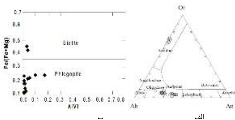
شکل ۳ الف. نمایش ترکیب فلدسپارهای سنگ‌های آتشفشانی ائوسن جنوب غرب چوپانان بر روی نمودار مثلثی An-Alb-Or [۱۴] ب. نمودار تقسیم‌بندی میکاهای سنگ‌های آتشفشانی ائوسن جنوب غرب چوپانان [۱۵].
