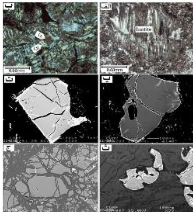
شکل ۵ الف) بافت بستایت؛ سرپانتین همراه با کانی های اپک به موازات کلیواژ پیروکسن (PPL)، ب) بافت شیشه ساعتی و کانی های لیزاردیت و کریزوتیل در پریدوتیت سرپانتینی شده (XPL)، پ، ت، ث) تصاویر SEM از اسپینل های منطقه مورد مطالعه، رنگ نسبتاً روشن در حاشیه و در امتداد شکستگی ها به دلیل تبدیل اسپینل به مگنتیت است، ج) تصویر SEM از بافت مش در الیوین.
