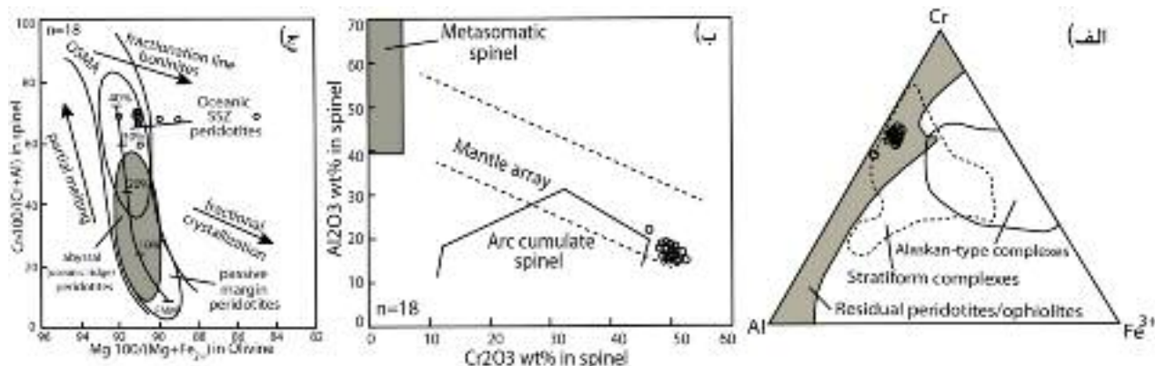
شکل ۸ الف) نمودار مثلثی Al-Cr-Fe 3+ در اسپینل پریدوتیت‌های سوره دال، محدوده کرومیتیت از [۱۵] و بقیه محدوده‌ها از [۱۶] است. ب) نمودار Cr 2 O 3 wt% در مقابل Al 2 O 3 wt% در اسپینل [۱۷]، نمونه‌های مورد مطالعه در محدوده شاخص گوشته‌ای واقع می‌شوند ج) Cr# اسپینل در مقابل Mg# الیون در پریدوتیت‌های سوره دال، نمونه‌ها در محدوده SSZ رسم شده‌اند. محدوده‌های abyssal peridotites, Fractionation line و OSMAs (oceanic ridge, oceanic SSZ, passive margin peridotites) از [۱۸، ۱۱]، هم‌چنین محدوده boninites [۱۹، ۱۲] می‌باشند.
