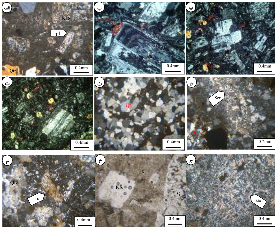
شکل ۵ الف- تصویر میکروسکوپی از ریولیت‌های منطقه (XPL) ب- تصویر میکروسکوپی از کوارتز مونزودیوریت پورفیری (XPL) پ- تصویر میکروسکوپی از پیروکسن هورنبلند دیوریت پورفیری، کانی هونبلند به کلریت دگرسان شده است. (XPL) ت- تصویر میکروسکوپی از آندزیت (XPL) ث- تصویر میکروسکوپی از رگه کوارتزی (XPL) ج- تصویر میکروسکوپی از دگرسانی آرژلیک-کوارتز-سرسیت-پیریت (XPL) ح- تصویر میکروسکوپی از دگرسانی سیلیس-آرژلیک-زمینه آرژیلی شده است و پیریت نیز به اکسیدهای آهن تبدیل شده است (XPL) خ- تصویر میکروسکوپی از دگرسانی سیلیس-آرژلیک (PL) چ- تصویر میکروسکوپی از دگرسانی آرژلیک پیشرفته (XPL) علائم اختصاری [۲۲] و Ser برای سرسیت، Alu برای آلونیت استفاده شده است.
