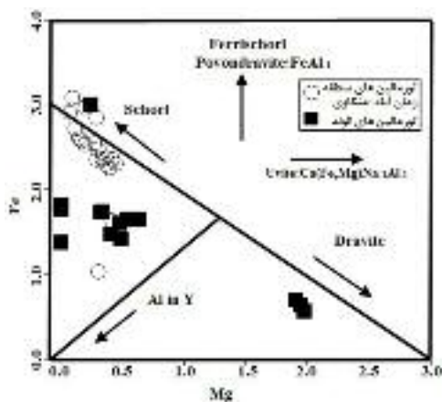
شکل ۸ موقعیت تورمالین‌های مورد بررسی روی نمودار Fe نسبت به Mg [۲].
