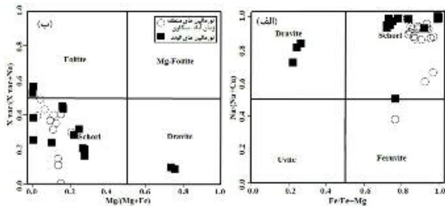
شکل ۵ موقعیت تورمالین‌های مورد بررسی (الف) روی نمودار Na/(Na+Ca) نسبت به Fe/(Fe+Mg) [۱۸] و (ب) روی نمودار X\text{-vac}/(X\text{-vac}+Na) نسبت به Mg/(Mg+Fe) [۱۹].
