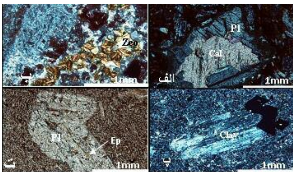
شکل ۷ الف) تبدیل پلاژیوکلاز به کلسیت در نور XPL (ب) حفرات پر شده با زئولیت در نور XPL (پ) تبدیل پلاژیوکلاز به کانی رسی در نور PPL (ت) تبدیل پلاژیوکلاز به اپیدوت در نور PPL، Ep: اپیدوت، Cal: کلسیت، Pl: پلاژیوکلاز، Zeo: زئولیت، Clay: کانی رسی).
