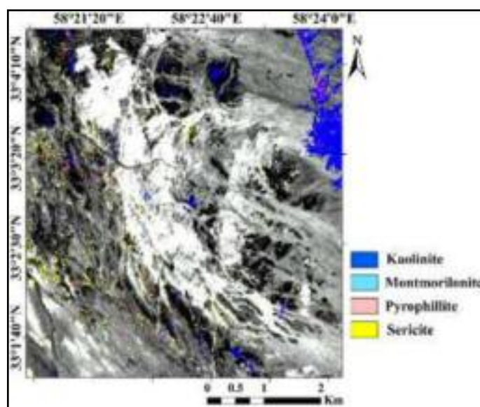
شکل ۳ تصاویر ماهواره‌ای آستر، که دگرسانی آرژیلیک بر روی آن بارزسازی شده است.
