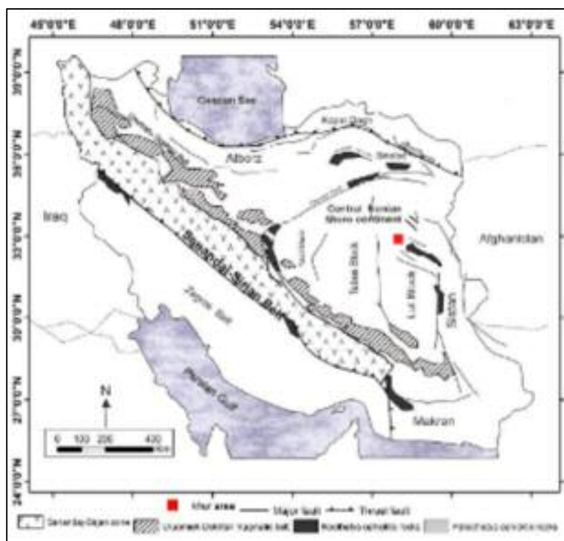
شکل ۱ موقعیت منطقه‌ی مورد بررسی در بلوک لوت [۳-۱].
