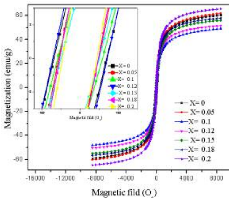
شکل ۵ حلقه‌های پسماند مغناطیسی نانو ذرات فریت Ni_{0.65}Zn_{0.35}Cu_xFe_{2-x}O_4 .
