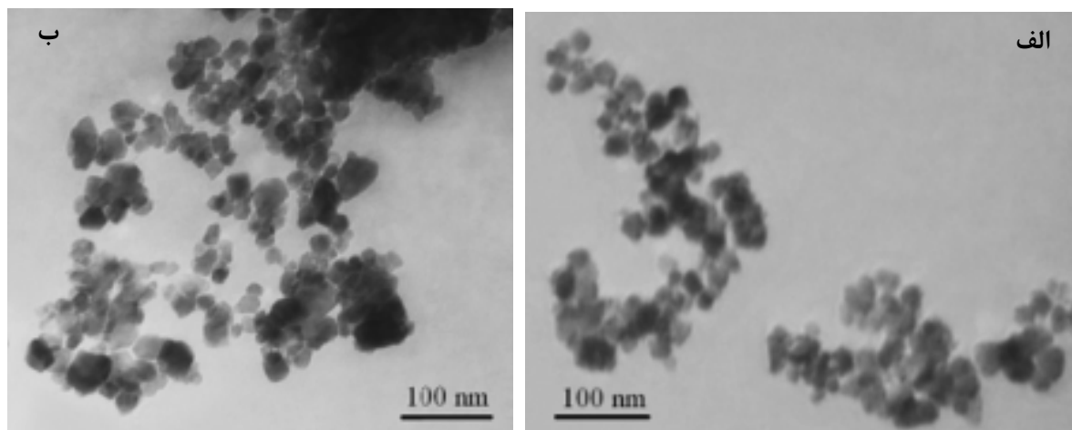
شکل ۴ تصاویر TEM (الف) Ni_{0.65}Zn_{0.35}Cu_{0.1}Fe_{1.9}O_4 و (ب) Ni_{0.65}Zn_{0.35}Cu_{0.18}Fe_{1.82}O_4 .
