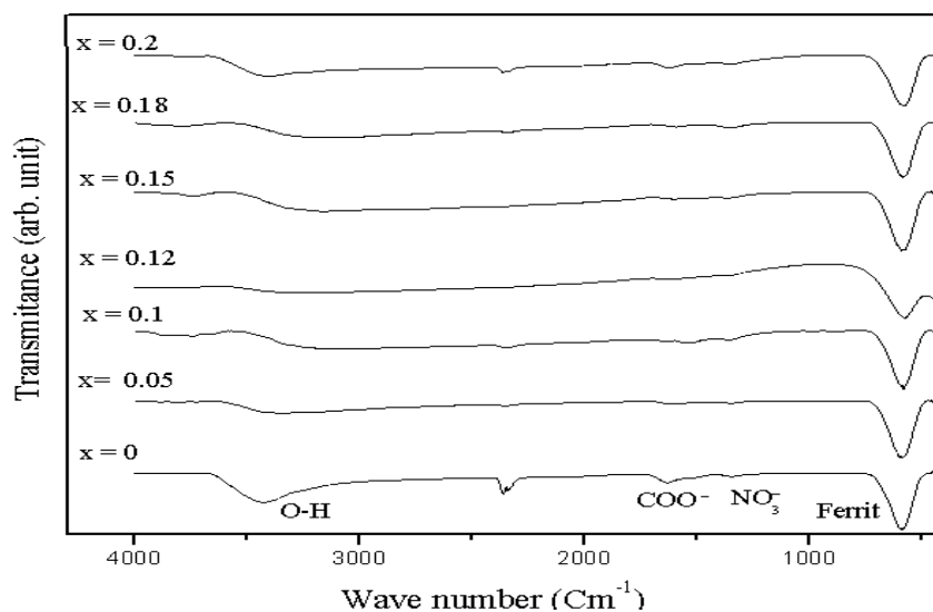
شکل ۲ طیف‌های فرسرخ نانو ذرات فریت Ni_{0.65}Zn_{0.35}Cu_xFe_{2-x}O_4 .
