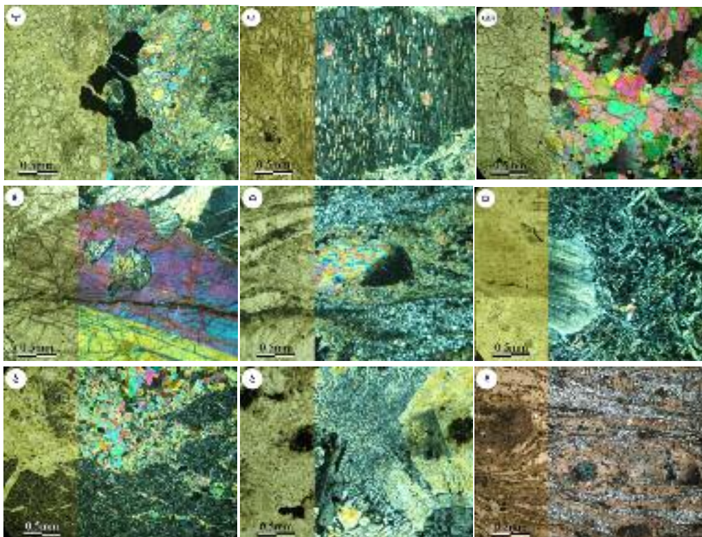
شکل ۲ تصاویر مقاطع میکروسکوپی در نور معمولی و قطبیده. (الف) نمونه هارزبورژیتی با شکنج در الیوین. (ب) تیغه‌های جدایشی کلینوپیروکسن در ارتوپیروکسن. (پ) بلورهای کروم اسپینل در نمونه‌های پریدوتیتی. (ت) بافت غربالی در سرپانتینیت‌ها. (ث) پیچ و تاب خوردگی نامتقارن ارتوپیروکسن در هارزبورژیت. (ج) درشت بلورهای کلینوپیروکسن و پلاژیوکلاز در گابروهای پگماتوئیدی. (چ) بلورهای کلینوپیروکسن در ماتریکس ریز بلور پلاژیوکلاز در گابروهای میلیونیتی. (ح) بافت گرافیکی ناشی از هم‌رشدی کوارتز و پتاسیم فلدسپار. (خ) نمونه‌ی میکروسکوپی اجزای دایکی.
