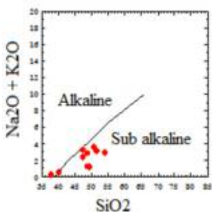
شکل ۷ نمودار قلیایی-سیلیس نمونه های مافیک و اولترامافیکی صحنه.
