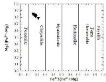
شکل ۳ ترکیب یونین سنگهای گابرویی بر پایه نمودار نسبت به Mg/(Fe^{2+}+Mg) .
