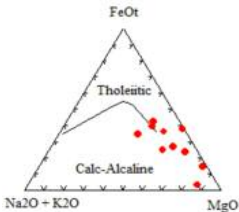
شکل ۸ نمودار AFM نمونه های مافیک و اولترامافیکی صحنه.
