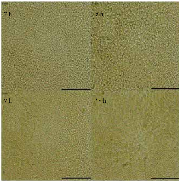
شکل ۷- تصاویر TEM آمیخته 30/70 PS/PVME حاوی ۲٪ نانوذرات A200 در زمان‌های مختلف جدایی فاز در دمای 110^\circ\text{C} (اندازه تمام خط‌های نشانه سیاه‌رنگ برابر 30 \mu\text{m} است).
