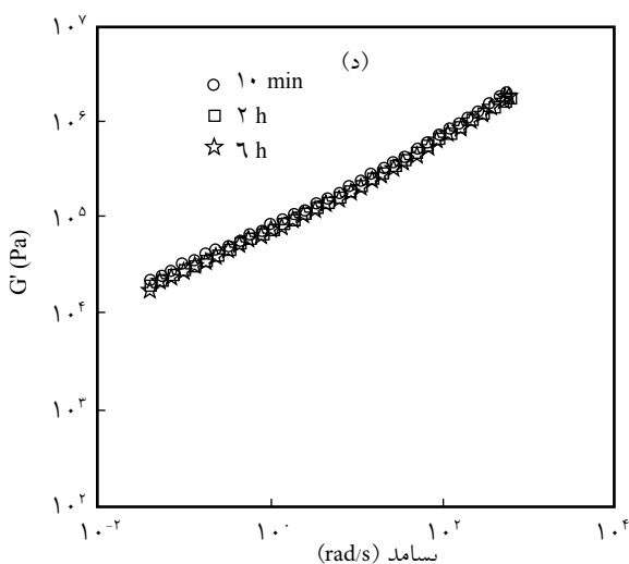
شکل ۹- آزمون پویس بسامد مدول کشسانی در زمان‌های مختلف جدایی فاز در دمای ۱۱۰°C برای آمیخته ۳۰/۷۰ PS/PVME با وجود مقادیر حجمی مختلف نانوذرات A200: (الف) ۰، (ب) ۰/۵٪، (ج) ۱٪ و (د) ۲٪.
