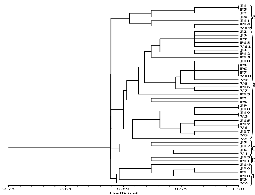
شکل ۴- گروه بندی ۴۹ جدایه F. culmorum بر اساس بیماریزایی با روش UPGMA و با استفاده از ضریب تشابه Nei and Li
