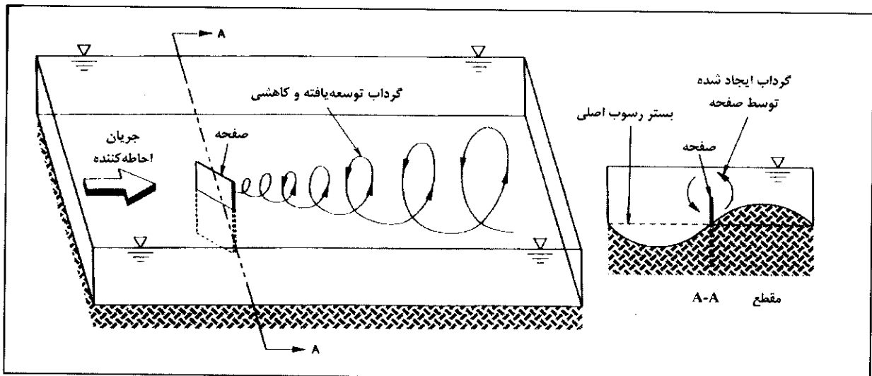
شکل شماره ۲- شیار آب شستگی ایجاد شده بر اثر صفحه مستغرق جلو دهانه آبیگر (Barkdoll, 1997)
