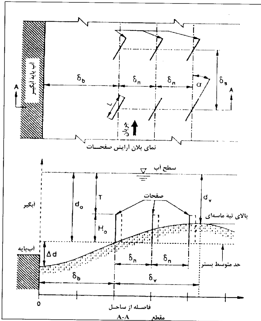
شکل شماره ۳- متغیرهای طراحی سیستم صفحات مستغرق (Wang et al., 1996)
