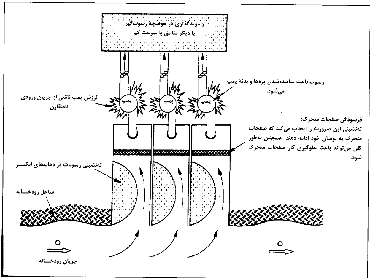
شکل شماره ۱- مشکلات ناشی از ورود رسوب به داخل دهانه آبیگر (Barkdoll, 1997)
