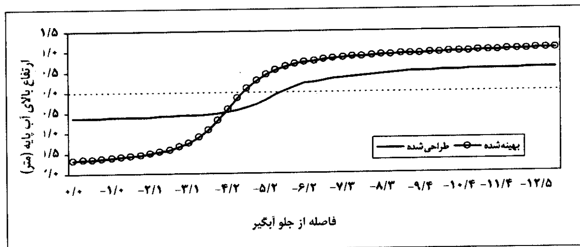
شکل شماره ۵- مقطع عرضی بستر جلو دهانه آبگیر DAEC در حالت طراحی شده و بهینه شده با روش جهات امکان پذیر
