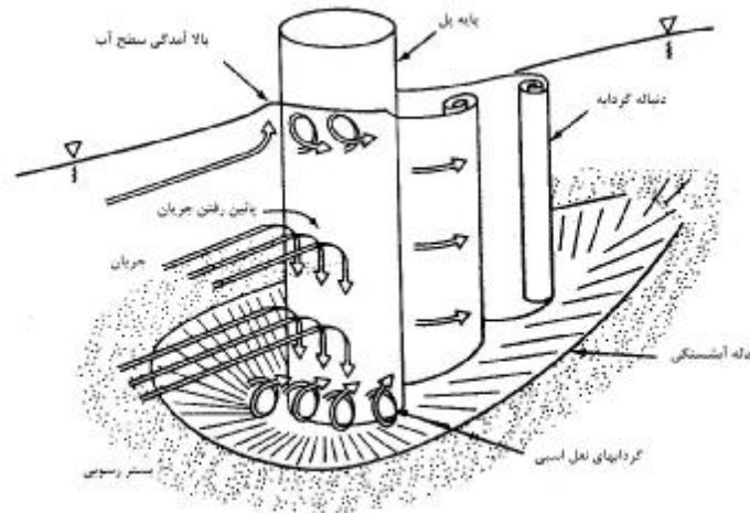
شکل ۱. الگوی جریان و حفره آبستگي موضعی اطراف یک پایه پل استوانه‌ای
