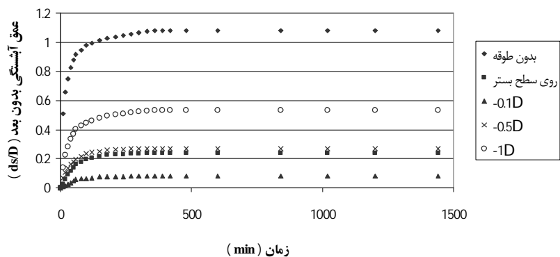
شکل ۷. تأثیر ارتفاع نصب طوقه نسبت به تراز بستر در مقایسه با پایه بدون طوقه در قطرهای مختلف روی آبشستگی
