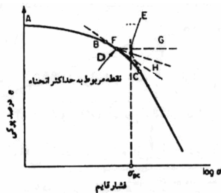
شکل ۲. یافتن تنش پیش‌تراکمی به روش کاساگران (۵).
