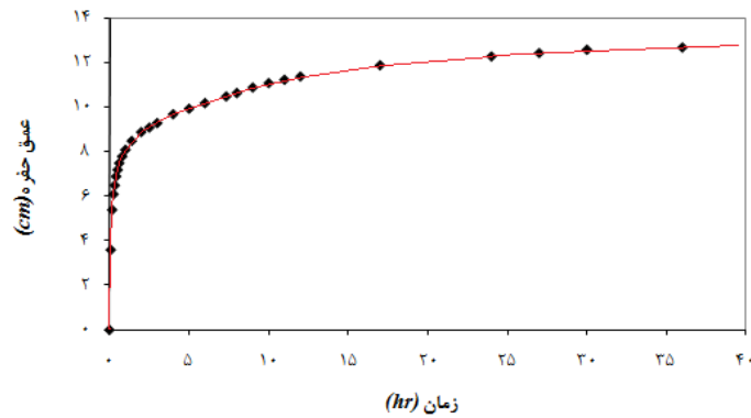
شکل ۳. نمودار توسعه زمانی آبستگی پایه بدون حفاظت.
