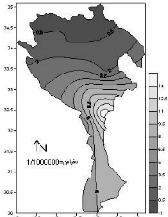
شکل ۳. نقشه ناحیه‌بندی شاخص Q_{7.10}
