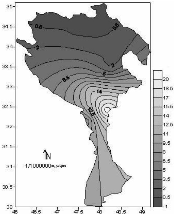
شکل ۵. نقشه ناحیه‌بندی شاخص Q_{3.10}
