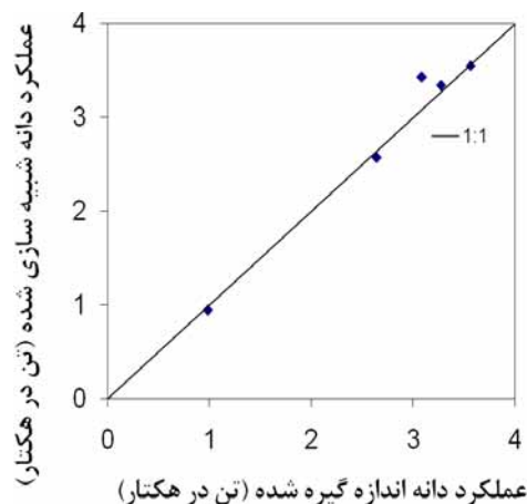
شکل ۴. مقادیر شبیه‌سازی و اندازه‌گیری شده محصول کلزا توسط مدل CRPSM با خط ۱:۱ محصول کلزا وارسته لیکورد سری داده‌های مستقل شعبانی و همکاران (۵)
