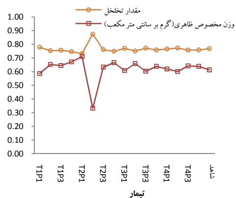
شکل ۱۵. مقایسه روند تخلخل و وزن مخصوص ظاهری برای ادوات مختلف خاک‌ورزی با دفعات مختلف پادلینگ
