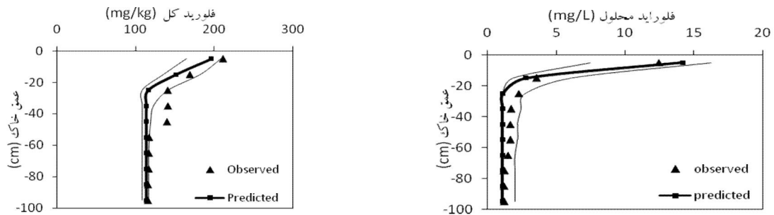
شکل ۳. غلظت فلوراید محلول و فلوراید کل شبیه سازی شده توسط نرم افزار HYDRUS-1D ۱۲۵ روز پس از افزودن نمک فلوراید سدیم در غلظت ۳۱۸ میلی گرم فلوراید در لیتر
