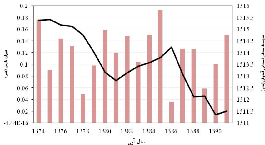
شکل ۷. هیدروگراف آبخوان سطحی زیرحوضه کوهپایه- سگزی همراه با بارش سالانه طی سال‌های ۱۳۷۴ تا ۱۳۹۱
