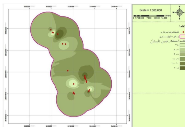
تصویر 3- نقشه پهنه‌بندی میانگین غلظت عنصر آرسنیک در منابع آب زیرزمینی دشت قهاوند در فصل تابستان
