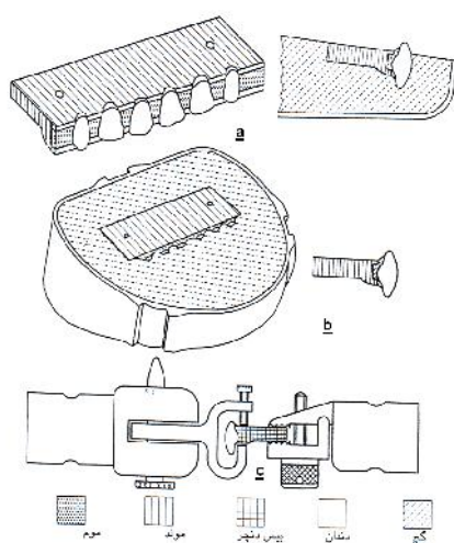
شکل ۴- قالب فلزی
