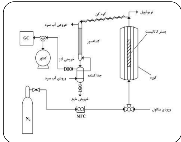
شکل ۱- نمایی از دستگاه آزمون راکتوری.
