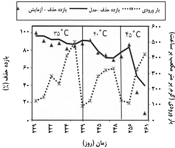
شکل ۴- مقایسه بازده حذف مدل و آزمایش در حالت بارگذاری پیوسته در دمای ۳۵ - ۴۵ درجه سانتیگراد.
