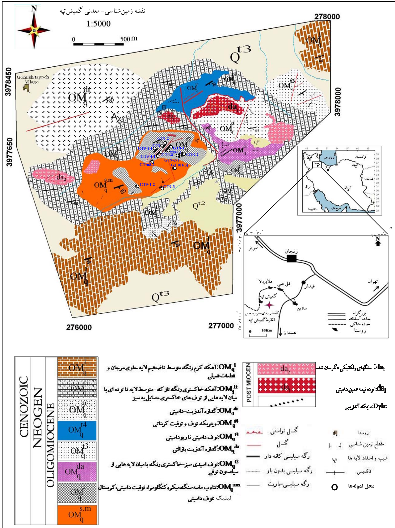
شکل ۱. موقعیت کانسار گمیش تپه در جنوب غربی زنجان و نقشه زمین‌شناسی - معدنی ۱:۵۰۰۰ [۲]. نتایج آنالیز نمونه‌های معدنی در جدول ۴ آورده شده است.
