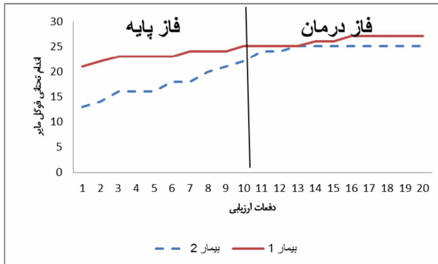
شکل 2- نمرات آزمون اندام تحتانی فوگل مایر بیماران
