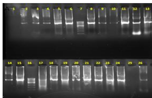
شکل ۳: (A) الکتروفورز RNAهای استخراج شده در روزهای جنینی جهت بررسی کیفی حضور باندهای ۲۸S و ۱۸S بر روی ژل آگارز، (B) الکتروفورز cDNAهای مزنسفالن مغز جوجه (روز ۱۹ جنینی) وزن GAPDH بر روی ژل آگارز جهت استفاده در Real time PCR چاهک ۱ مربوط به ژن GAPDH، چاهک ۲ مربوط به نشانگر و چاهک ۳ مربوط به ژن SALL4 می‌باشد.
