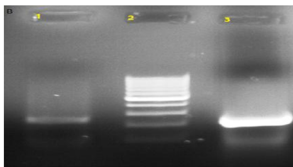
شکل ۳: (A) الکتروفورز RNAهای استخراج شده در روزهای جنینی جهت بررسی کیفی حضور باندهای ۲۸S و ۱۸S بر روی ژل آگارز، (B) الکتروفورز cDNAهای مزنسفالن مغز جوجه (روز ۱۹ جنینی) وزن GAPDH بر روی ژل آگارز جهت استفاده در Real time PCR چاهک ۱ مربوط به ژن GAPDH، چاهک ۲ مربوط به نشانگر و چاهک ۳ مربوط به ژن SALL4 می‌باشد.
