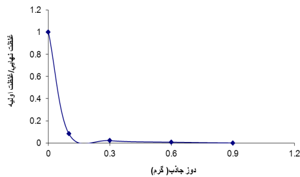
نمودار ۷. رابطه بین میزان جذب با مقدار دوز جاذب
