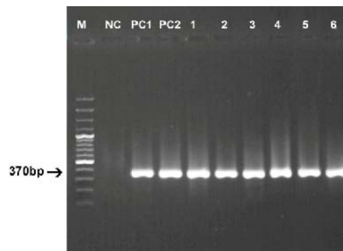
شکل ۱) تصویر الکتروفورز ژل آگارز مربوط به جنس لیستریا. M: مارکر ۱۰۰ جفت بازی، NC: کنترل منفی، PC1: کنترل مثبت لیستریای مونوسیتوژنز، PC2: کنترل مثبت لیستریای ایوانوای، ۱ تا ۶: ایزوله‌های مثبت برای جنس لیستریا
