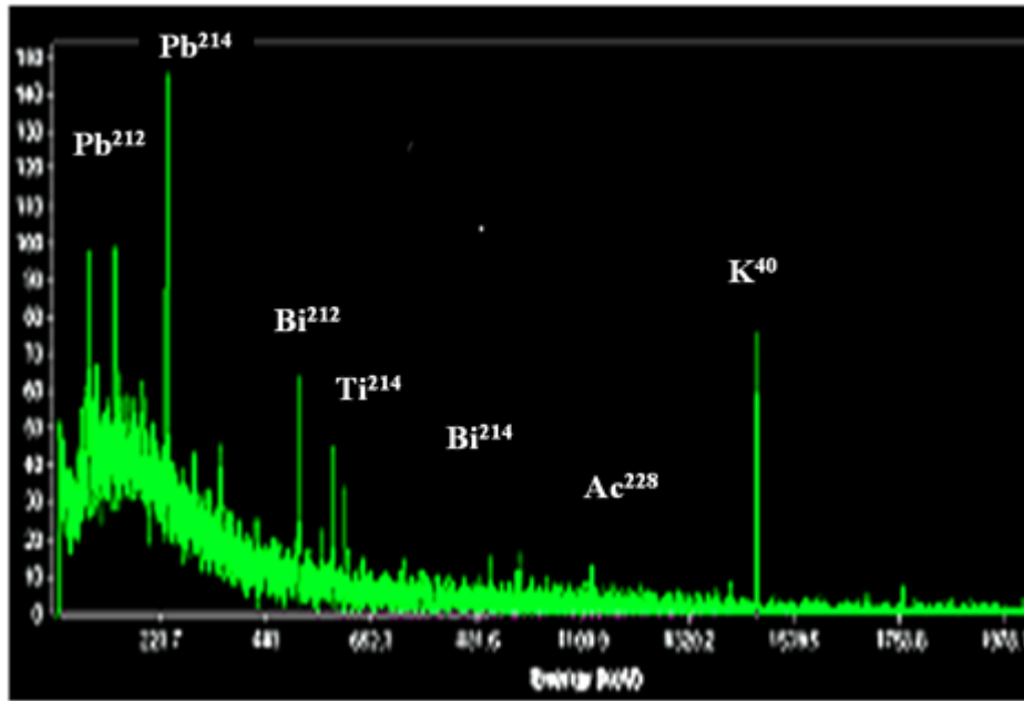
شکل ۲. \gamma اسپکتروم از آئروسول‌های جمع آوری شده
