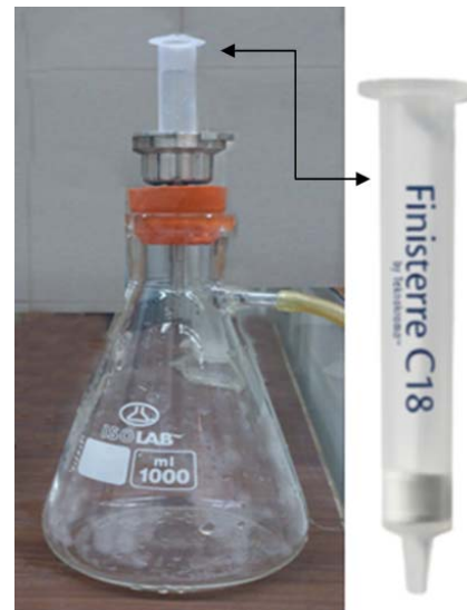
شکل ۲. ستون فاز جامد و نحوه استفاده از آن
