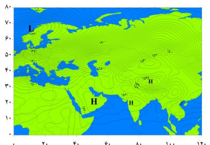
شکل (۱۱) الگوی چهارم 850hpa
