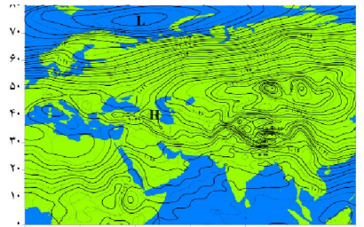
شکل (۳) الگوی دوم SLP
