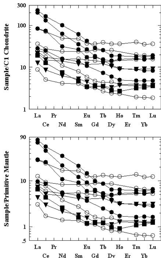
شکل ۱۹- الگوهای عناصر نادر خاکی به‌هنجار شده نسبت به کندریت و گوشته اولیه (Sun and McDonough, 1989).
