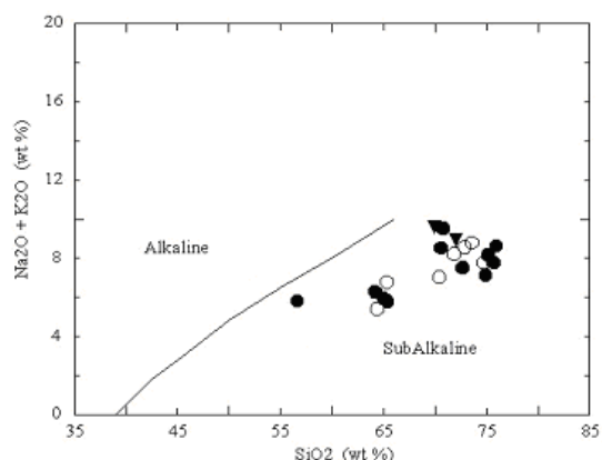
شکل ۱۵- ماگمای سازنده کمپلکس گرانیتوئید طبق Barager و Irvine (۱۹۷۱) ساب‌آلکان است. نمادها مانند شکل ۱۰ هستند.
