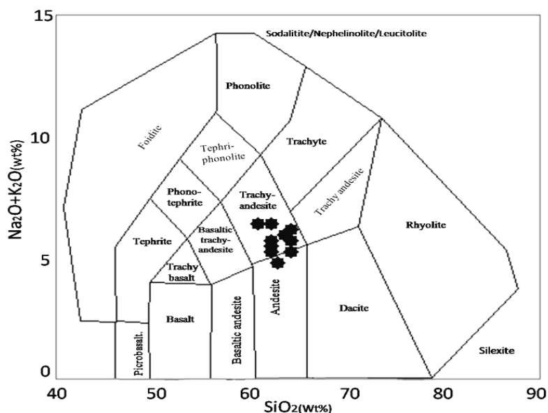
شکل ۵- نمودار رده‌بندی شیمیایی بر حسب مجموع آکالی‌ها (Na 2 O+K 2 O) در برابر SiO 2 (Middlemost, 1994)
