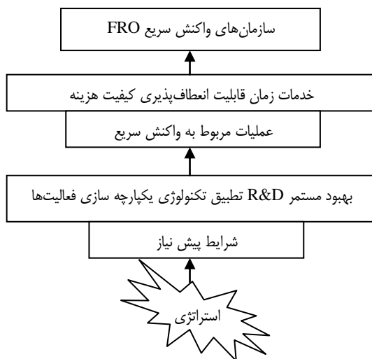
شکل ۲. الگوی ردفورد
