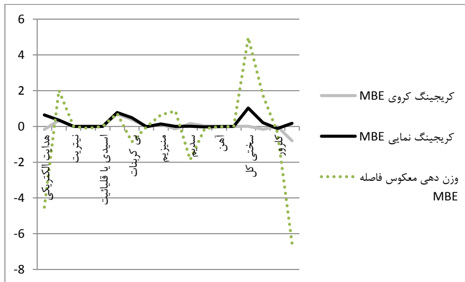
شکل ۴- چگونگی مقادیر MBE متغیرهای مختلف در روش‌های درون‌یابی IDW و کریجینگ با توابع نمایی و کرومی
