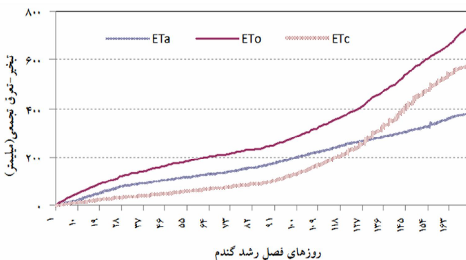
شکل 7- تبخیر- تعرق تجمعی (مرجع، استاندارد و واقعی) در مزارع تحت کشت گندم دشت آزادگان در فصل زراعی 1387-1386
