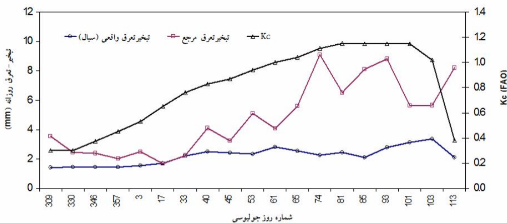
شکل 5- تغییرات ضریب گیاهی، تبخیر - تعرق واقعی و مرجع در مزارع تحت کشت گندم دشت آزادگان در طی فصل زراعی 1386-1387
