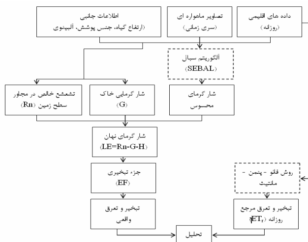
شکل 4- مراحل مختلف محاسبه تبخیر - تعرق واقعی با بکارگیری الگوریتم سبال (به نقل از پورمحمدی، 1388)
