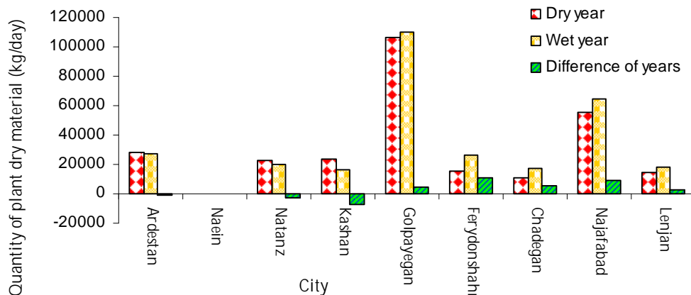
شکل ۱۰- مقایسه تغییرات میزان ماده خشک گیاهی در دو سال خشک (۲۰۰۰-۲۰۰۱) و تر (۲۰۰۴-۲۰۰۵) Fig. 10- Comparison of quantity of plant dry material in 2000-2001 dry and 2004-2005 wet years
