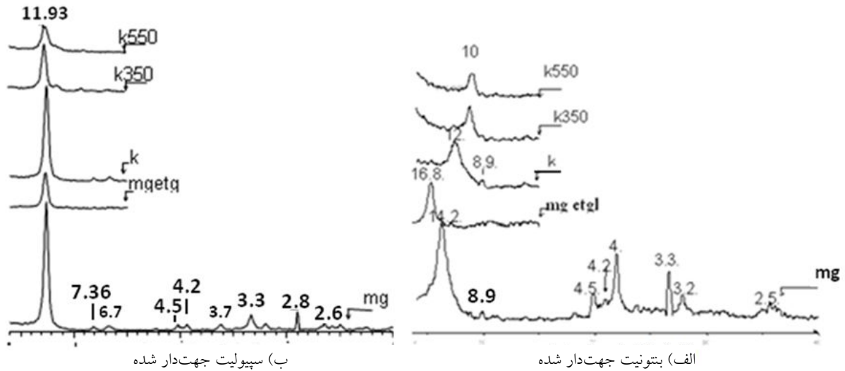
شکل ۲. دیفرکتوگرام اشعه ایکس نمونه‌های جهت‌دار شده بنتونیت (الف) و سپیولیت (ب)
