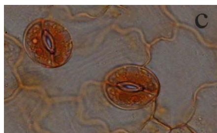
شکل ۲- تغییرات میزان گشودگی دهانه روزنه (ob: 100) در اپیدرم فوقانی در گیاه پرپوش ۷۰ روزه. (a) میزان گشودگی دهانه روزنه گیاه شاهد (هوگلند کامل محتوی کلات آهن)، (b) میزان گشودگی دهانه روزنه گیاه تحت غلظت ۰ \mu\text{l} نانوذرات اکسید آهن و (c) میزان گشودگی دهانه روزنه گیاه تحت غلظت ۳۰ \mu\text{l} نانوذرات اکسید آهن.
