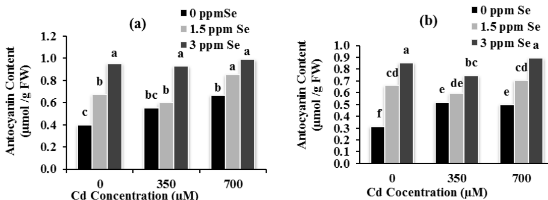
شکل ۴- اثر متقابل تیمار سلینیوم و کادمیوم بر محتوای آنتوسیانین در رقم کویر (a) و رقم روشن (b). مقایسه میانگین‌ها بر اساس آزمون دانکن و با سه تکرار انجام شد. حروف یکسان بیانگر عدم اختلاف معنی دار در سطح P \leq 0.05 است.
