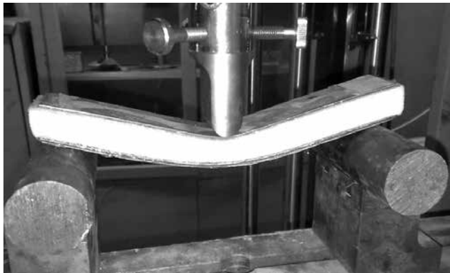
شکل ۱- نمونه زیر بارگذاری خمش سه نقطه‌ای.
