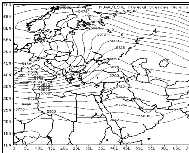
شکل ۳ نقشه مرکب الگوی اول در سطح زمین (سمت راست) و در تراز ۵۰۰ هکتوپاسکال (سمت چپ)
