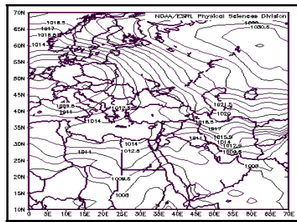
شکل ۳ نقشه مرکب الگوی اول در سطح زمین (سمت راست) و در تراز ۵۰۰ هکتوپاسکال (سمت چپ)
