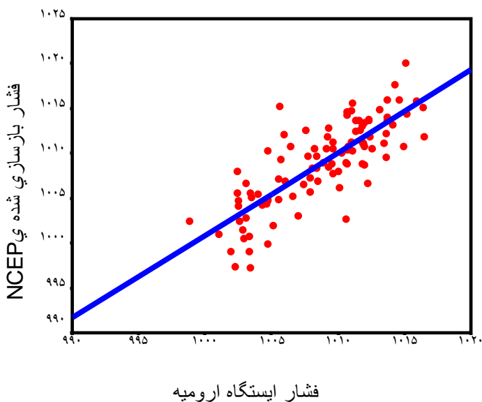
شکل ۲ نمودار پراکنش داده‌های فشار ایستگاه ارومیه و نزدیک‌ترین تلاقی NCEP همراه با برازش خط بهینه
